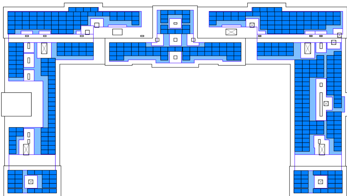
Abbildung 89: Mögliche Flächennutzung für Photovoltaik am Dach der Direktion Anteil der PV-Modulfläche an der gesamten Dachfläche: 37% (Quelle: Schöberl & Pöll GmbH)
