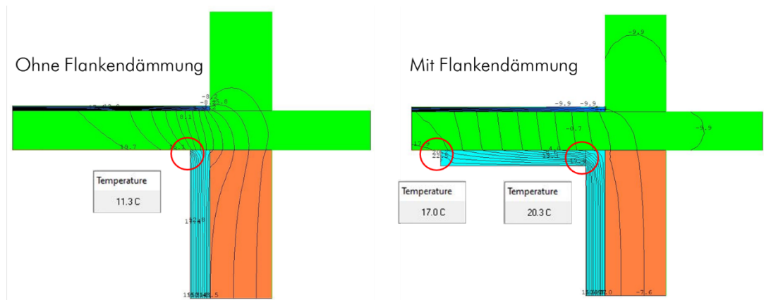
Abbildung 67: Vergleich des Isothermenverlaufs im Bereich der aufgesetzten Attika bei der Variante ohne Flankendämmung (links) und der optimierten Variante mit Flankendämmung (rechts)
