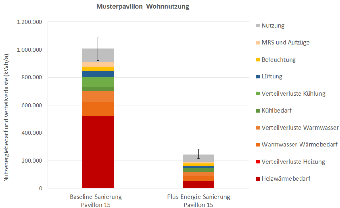
Abbildung 79: Nutzenergiebedarf und Verteilverluste - Pavillon 15, Wohnnutzung (Quelle: Schöberl & Pöll GmbH)
