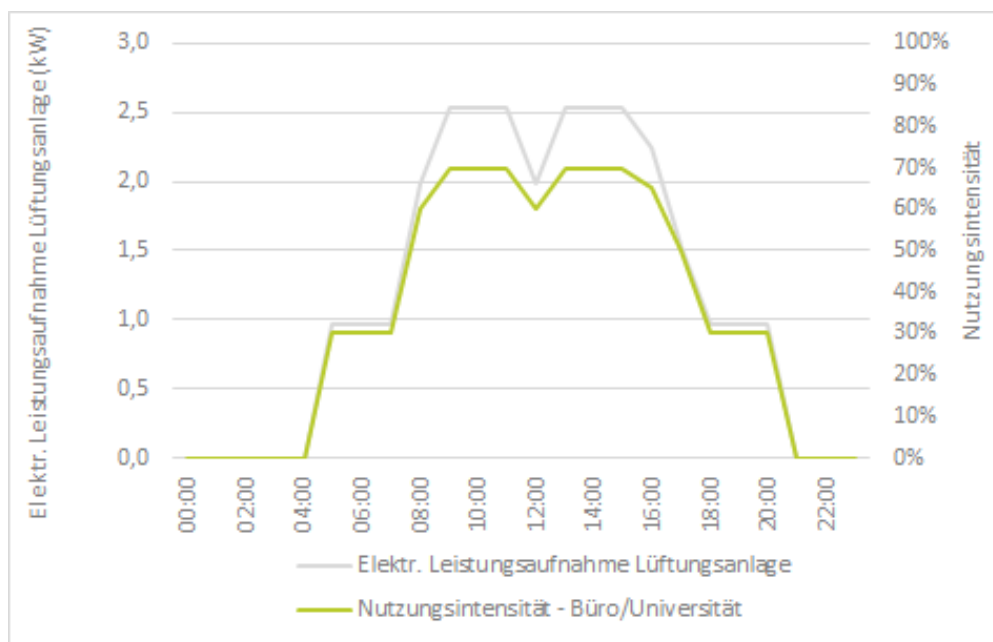
Abbildung 71: Elektrische Leistungsaufnahme Lüftungsanlage und Nutzungsintensität – Büro/Universität – Plus-Energie-Sanierung
