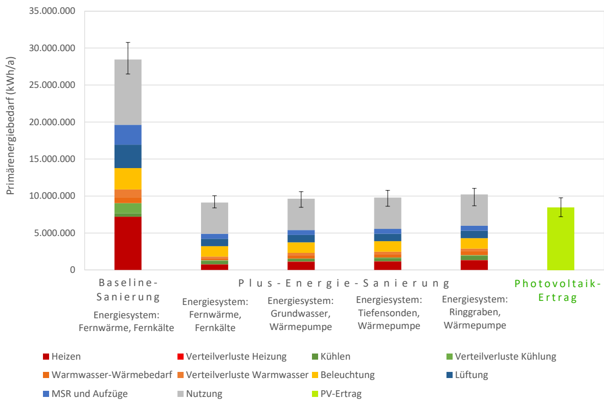
Abbildung 98: Primärenergiebilanz Otto-Wagner-Areal Gesamt mit allen untersuchten Geothermie-Systemen, inklusive Nutzung (Quelle: Schöberl & Pöll GmbH)
