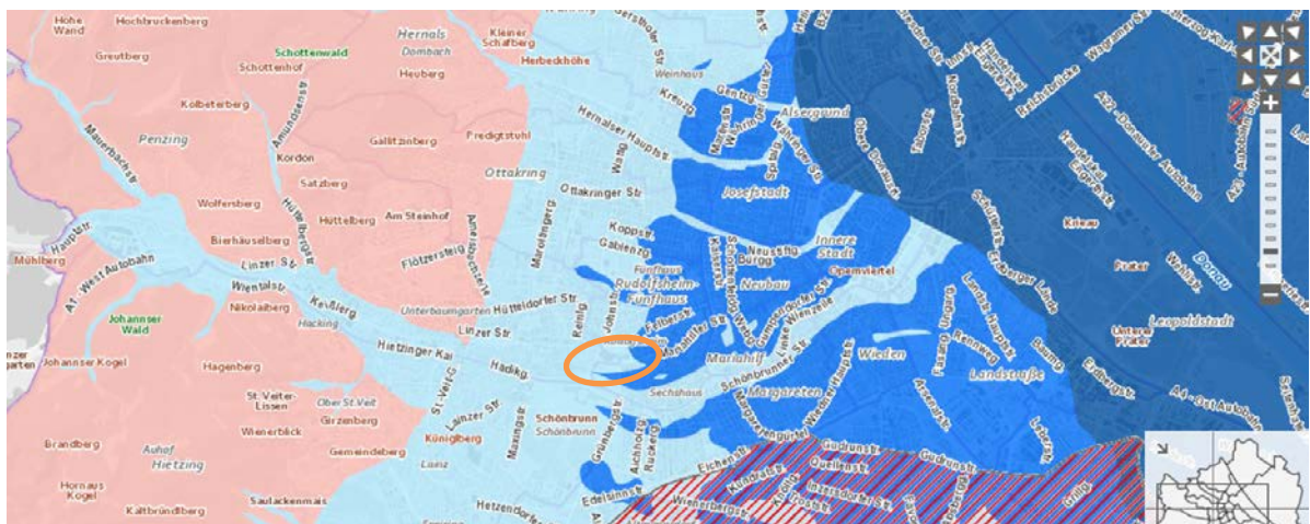
Abbildung 48: Thermische Grundwassernutzung laut Erdwärmepotenzialkataster der Stadt Wien 14
