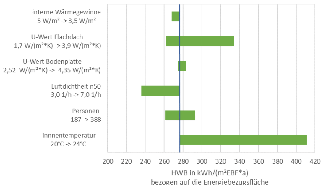
Abbildung 42: Sensitivitätsanalyse mit Passivhaus-Projektierungspaket (bezogen auf die Energiebezugsfläche). Die blaue Markierung stellt den Heizwärmebedarf unter Berücksichtigung der Basisannahmen dar. Die für die jeweiligen Parameter angegebenen Werte auf der Achsenbezeichnung der y-Achse sind immer von links nach rechts zu lesen, der erste Wert bedingt den niedrigsten Heizwärmebedarf und der zweite Wert den höchsten Heizwärmebedarf. Quelle: Schöberl & Pöll GmbH
