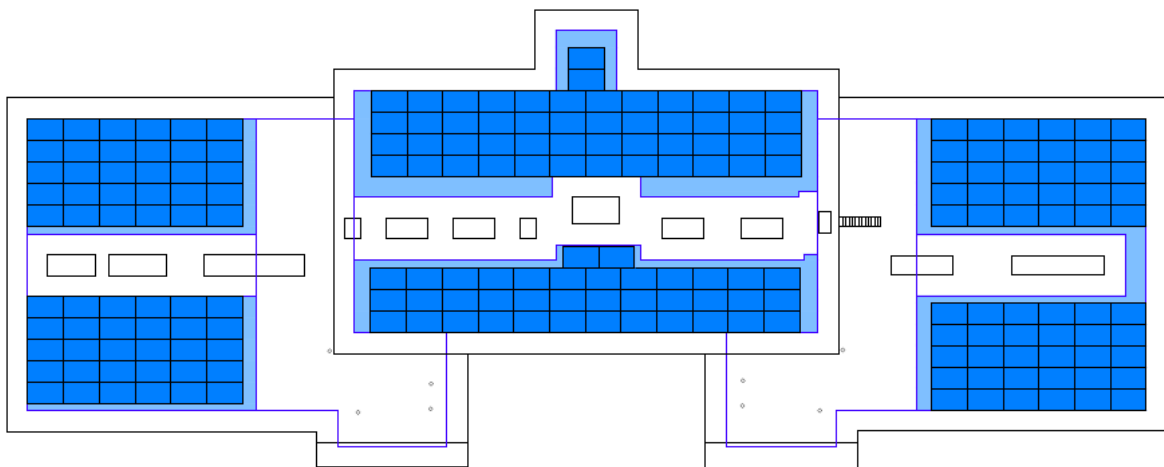
Abbildung 87: Mögliche Flächennutzung für Photovoltaik am Dach des Pavillon 10. Anteil der PV-Modulfläche an der gesamten Dachfläche: 39% (Quelle: Schöberl & Pöll GmbH)
