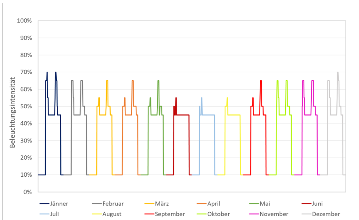
Abbildung 57: Simulierte Beleuchtungsintensität im Jahresverlauf für Büronutzung
