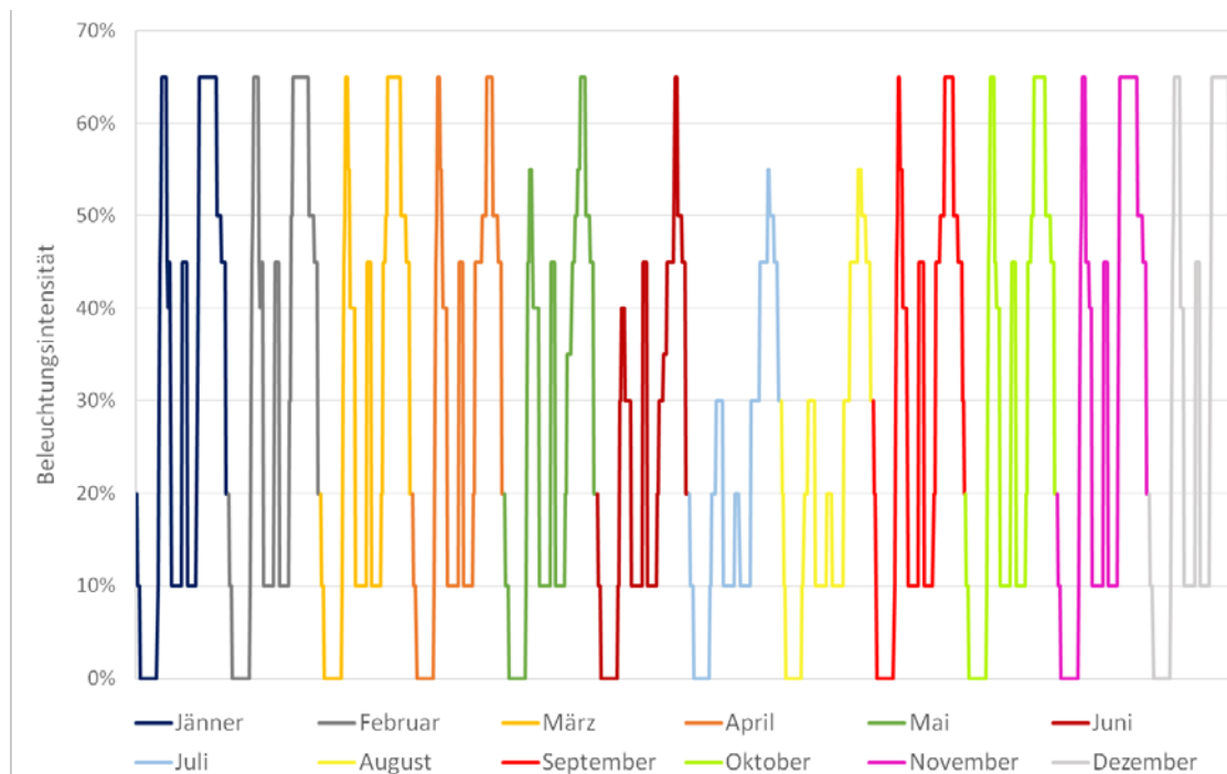
Abbildung 61: Beleuchtungsintensität im Jahresverlauf für Wohnnutzung
