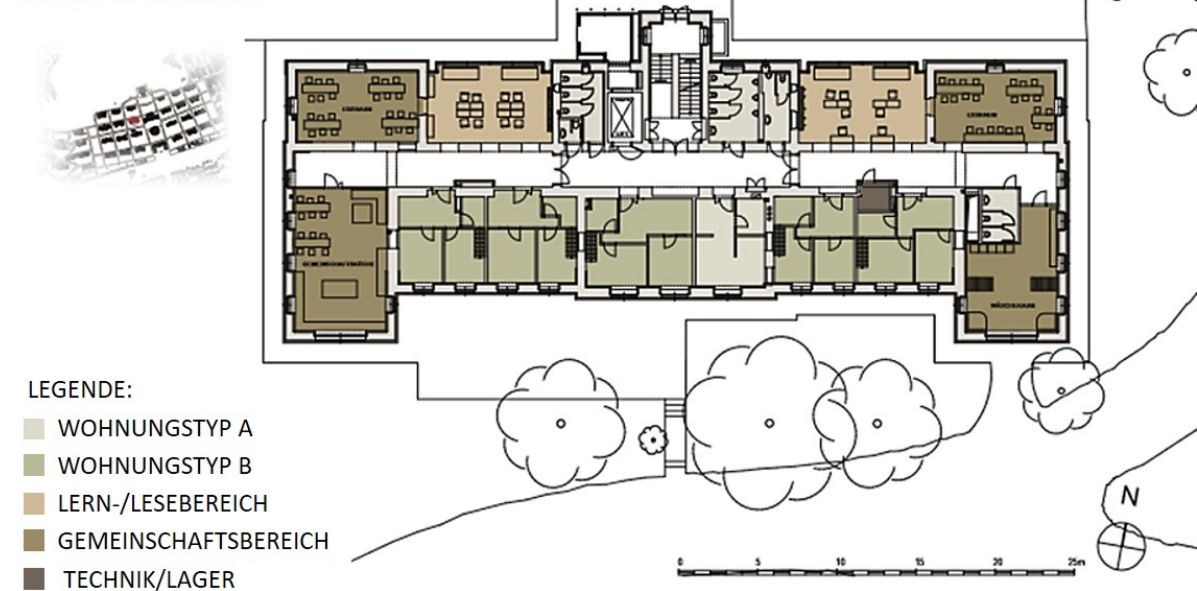
Abbildung 36: „Green Beetween“, Vorschlag für Umnutzung und Umbau von Pav. 13 für studentisches Wohnen, Erdgeschoß, Haas/Schmiedbauer (TU Wien, Entwerfen SS 2020, Organisation und Leitung: Karin Stieldorf)
