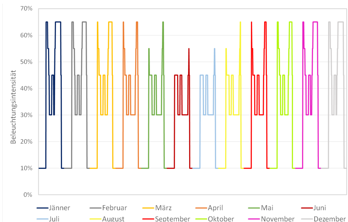
Abbildung 63: Beleuchtungsintensität im Jahresverlauf für Sondernutzung
