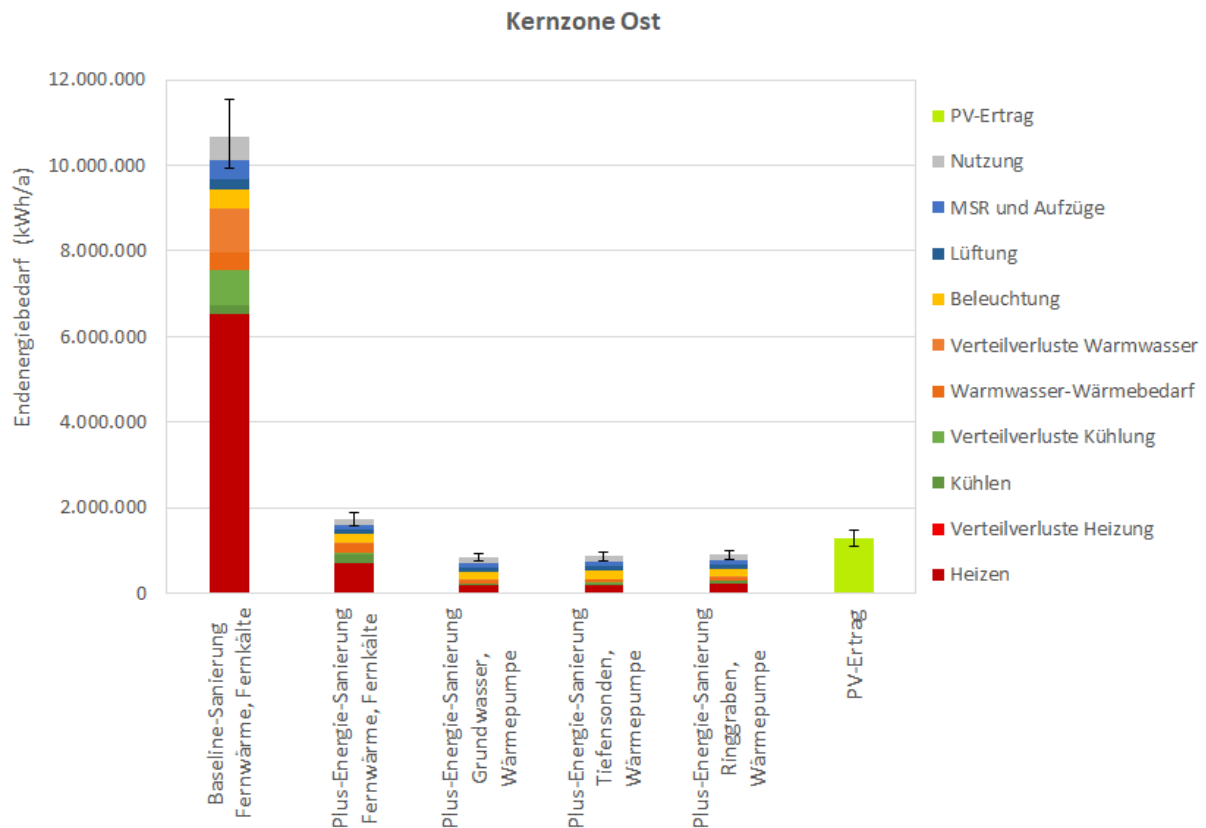
Abbildung 94: Endenergiebilanz Kernzone Ost (Quelle: Schöberl & Pöll GmbH)
