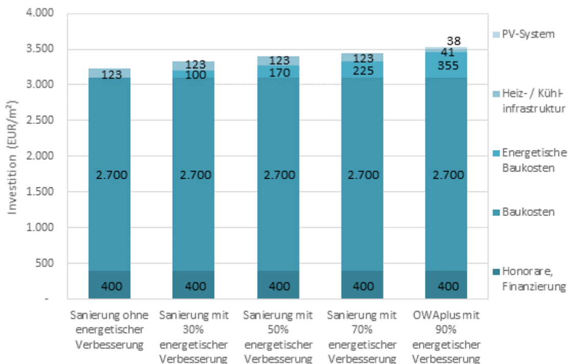
Abbildung 103: Gegenüberstellung der Investitionskosten je Sanierungsvariante (Quelle: LANG consulting)
