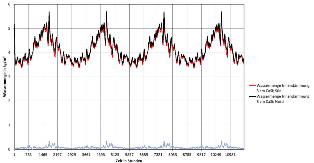
Abbildung 48: Gegenüberstellung der Wassermenge in \text{kg}/\text{m}^3 in der Innendämmung bei Nord- und bei Südorientierung
