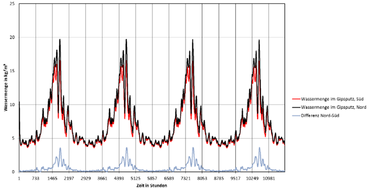
Abbildung 47: Gegenüberstellung der Wassermenge in \text{kg}/\text{m}^3 im Gipsputz bei Nord- und bei Südorientierung
